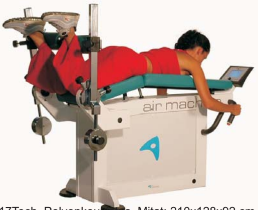
917Tech. Polvenkoukkaus. Mitat: 210x128x92 cm. Max.vastus: 60 kg/kahva. Liikelaajuuden rajoittimet. Tyynyjen ja vastapainojen säädöt. Penkin kulman säätö.
