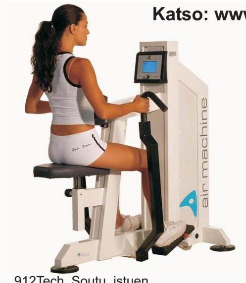
912Tech. Soutu, istuen. Mitat: 134x134x100 cm. Max. Vastus 60 kg. Säätävät istuin ja rintatuki.
